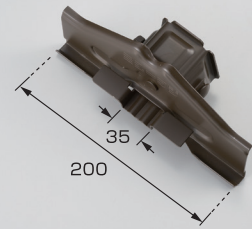
H-3 ニューフジ三晃式中
