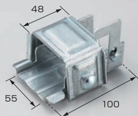
A-11 マナスル林式55mm
