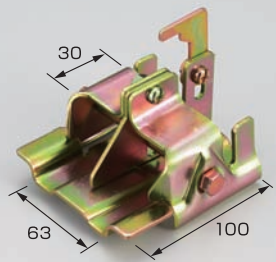
A-17 スノーストップ葺替用63mm
