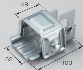
A-12 マナスル林式耳巻53mm
