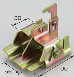
A-16 スノーストップ葺替用56mm
