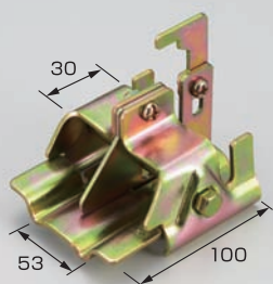
A-15 スノーストップ葺替用53mm
