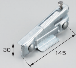
TA-2 立平用アンクル止 シャトル
