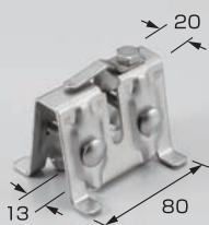
SH-12 NFハゼアングル止
