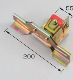
Y-32 スノーストップAT 小 アングル止付
