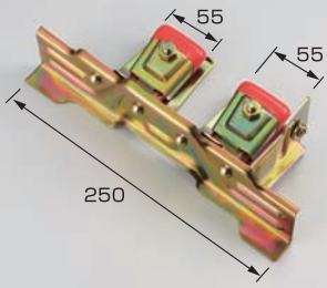
Y-30 スノーストップATW アングル止付
