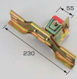
Y-31 スノーストップAT 中 アングル止付
