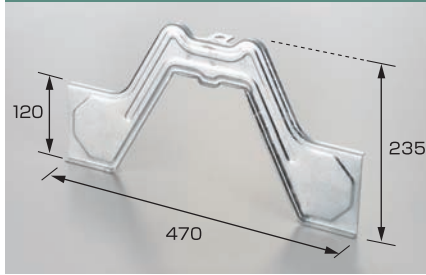
SH-4 SHハゼⅡ型羽根 ハゼ500
