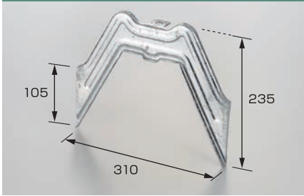
SH-3 SHハゼⅠ型羽根 ハゼ333
