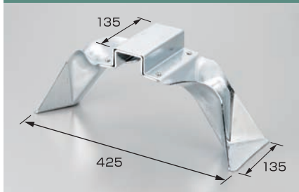
SH-7 スノーバレー角ハゼ2型用
