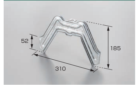
SH-5 SHハゼⅢ型羽根 ハゼ600
