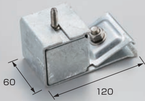
PV-1 平葺用PV金具
