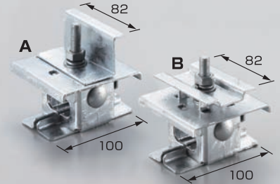
PV-3 ハゼ用PV金具 丸ハゼ
