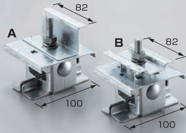
PV-2 ハゼ用PV金具 角ハゼ
